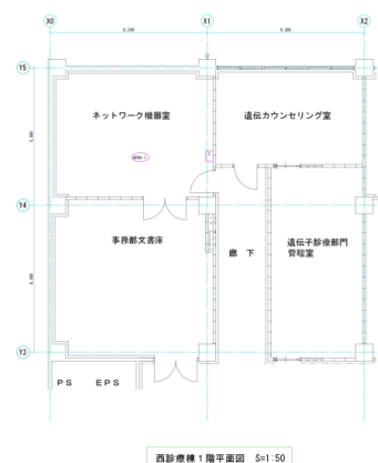
西診療棟1階平面図 S#1.50
